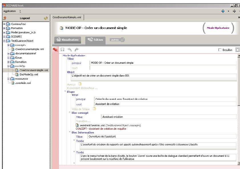
Figure 2 : Copie d'écran de l'éditeur de contenu dans SCENARIchain3 (ici un mode opératoire pour créer un document dans Business Object)
